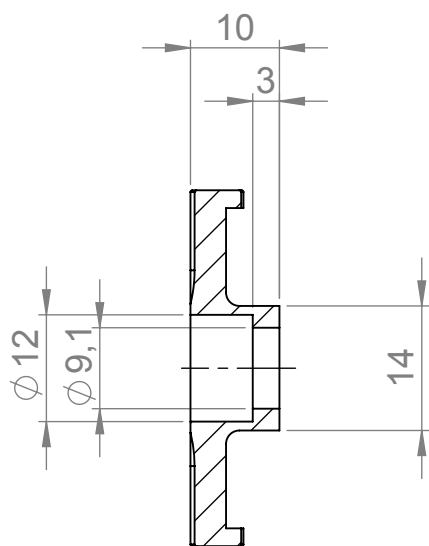
SCHNITT A-A
