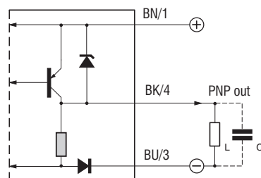
PNP output
