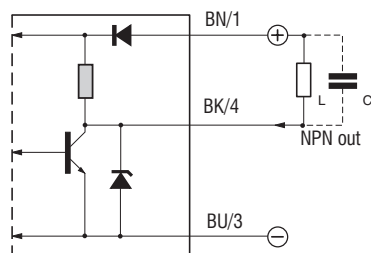
NPN output
