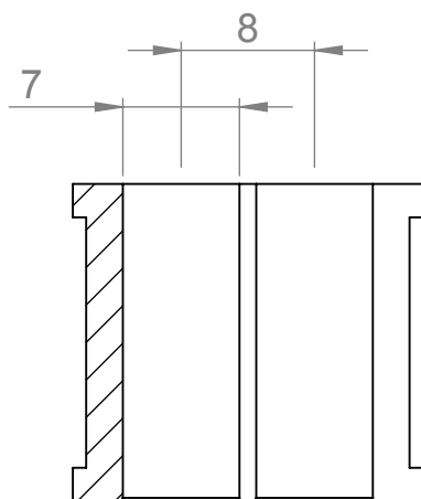
SCHNITT A-A
