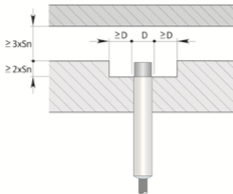
Montaggio sporgente
